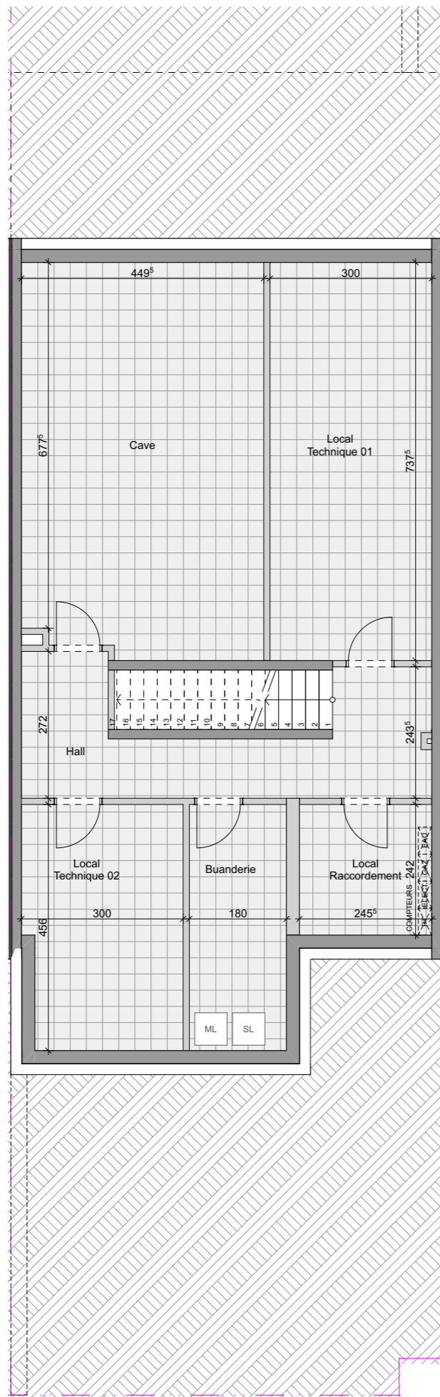
SOUS-SOL 1:100
