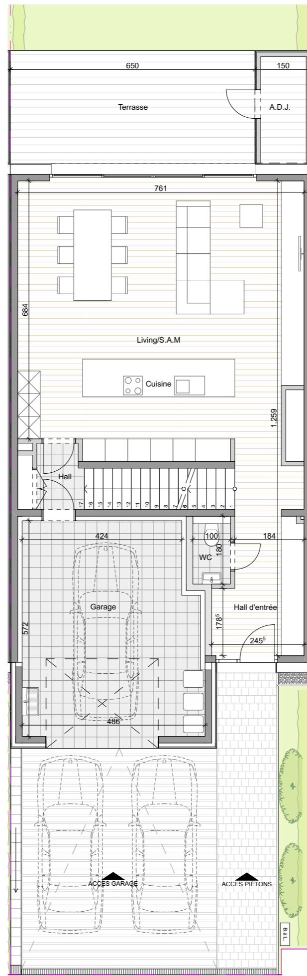
REZ-DE-CHAUSSEE 1:100
