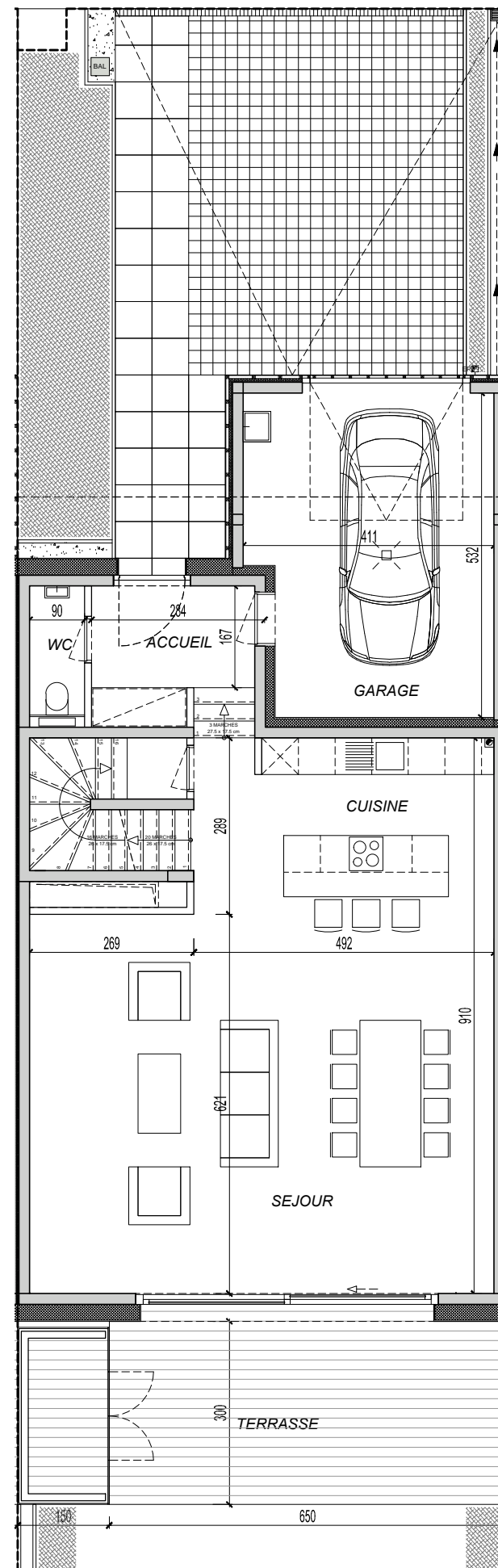
REZ-DE-CHAUSSEE 1/100
