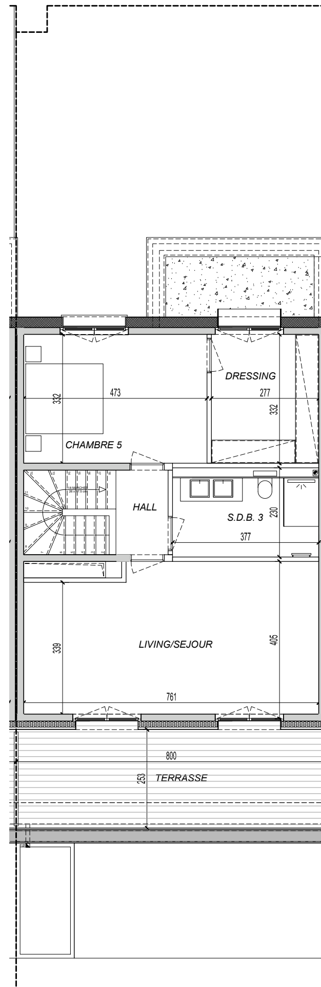
RETRAIT 1/100
