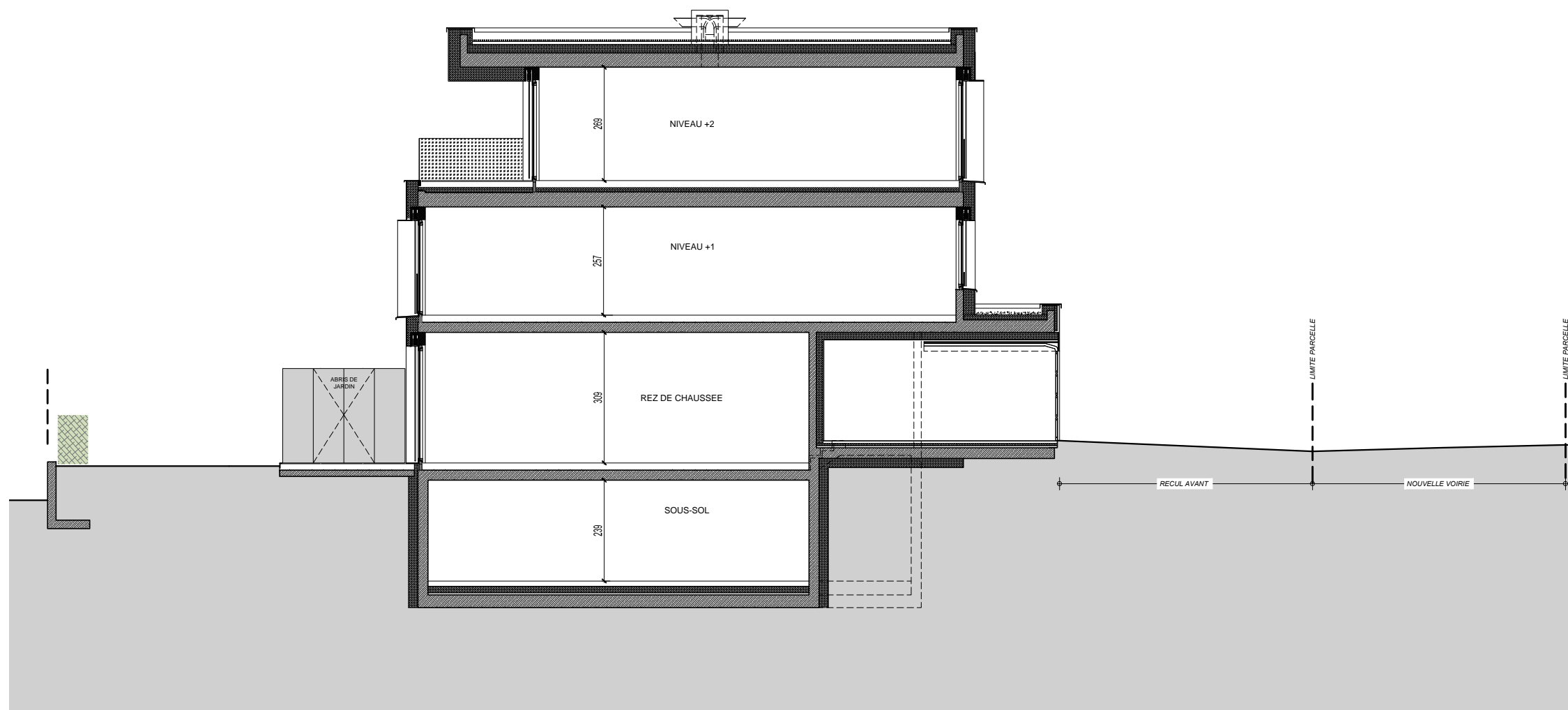
COUPE 1/125
