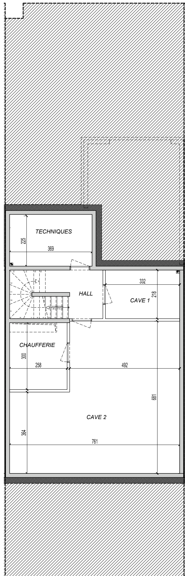
SOUS-SOL 1/100
