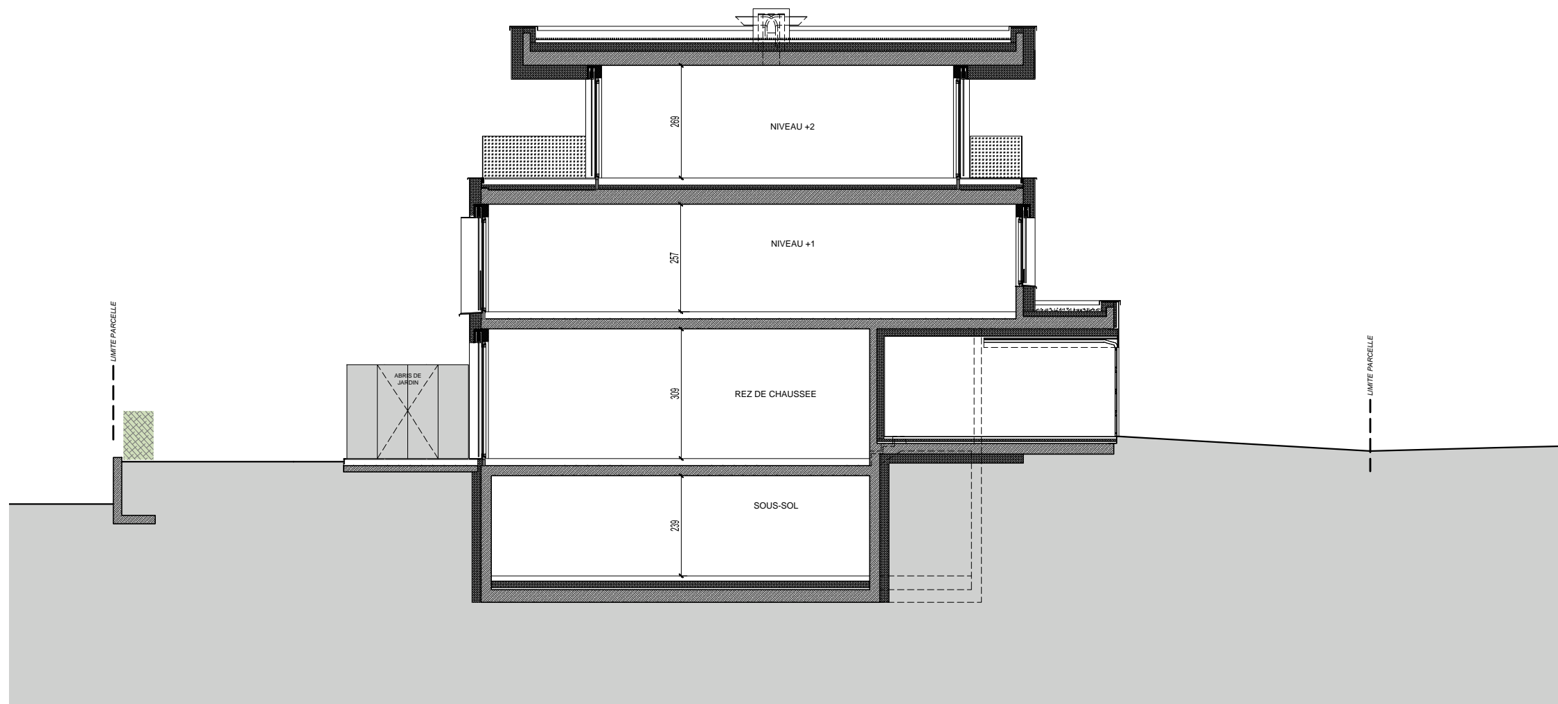
COUPE 1/100
