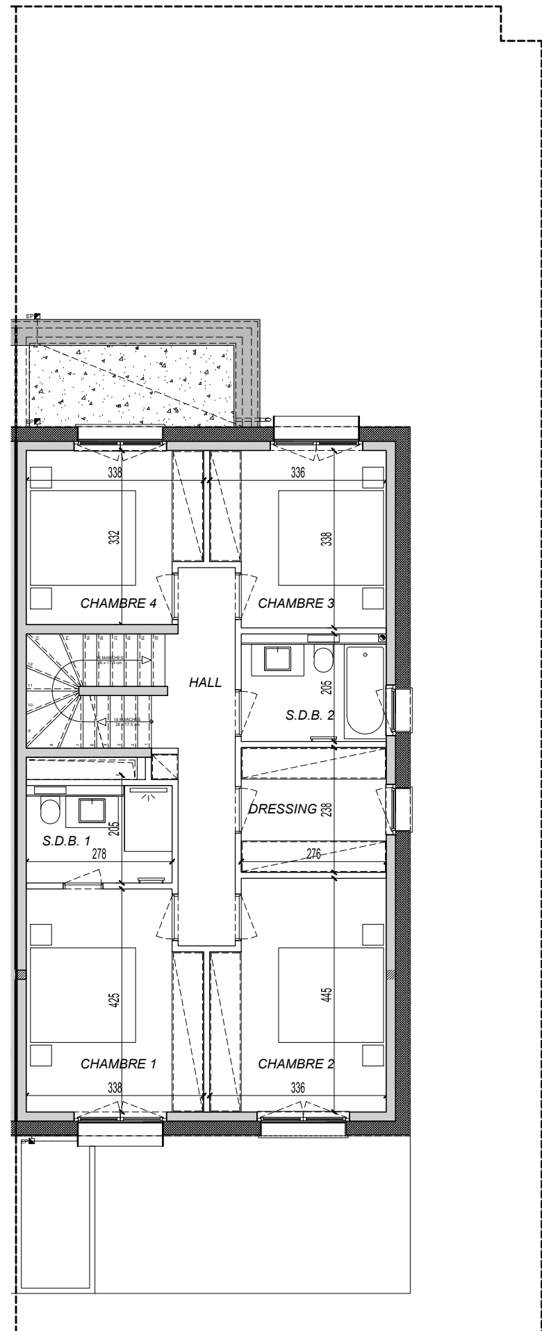
ETAGE 1/100
