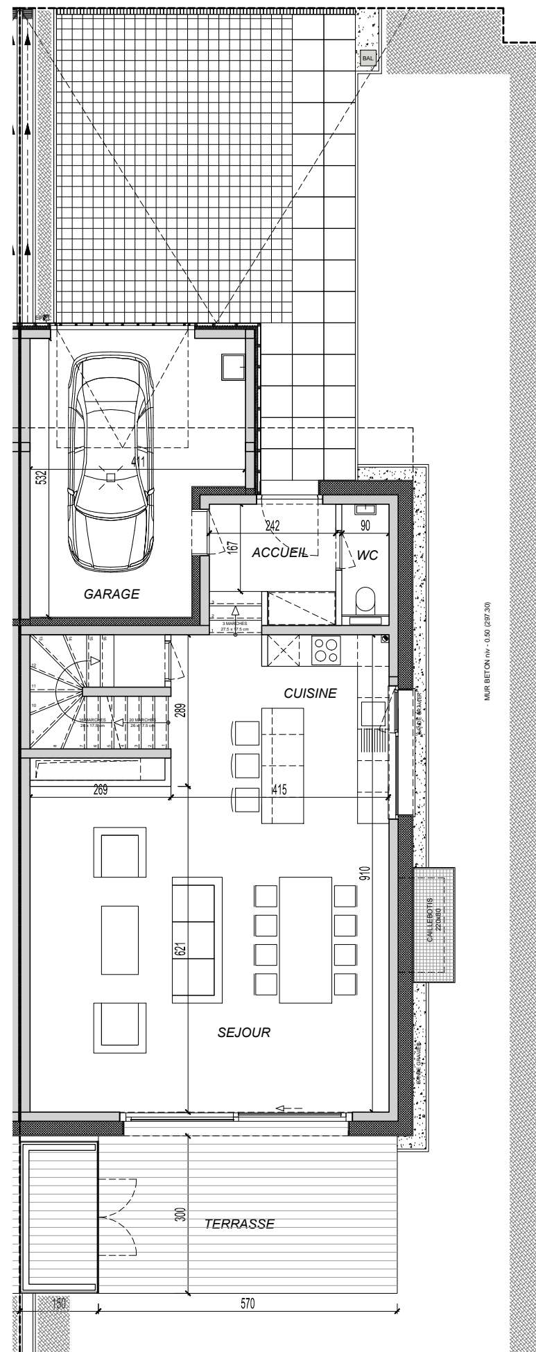
REZ-DE-CHAUSSEE 1/100
